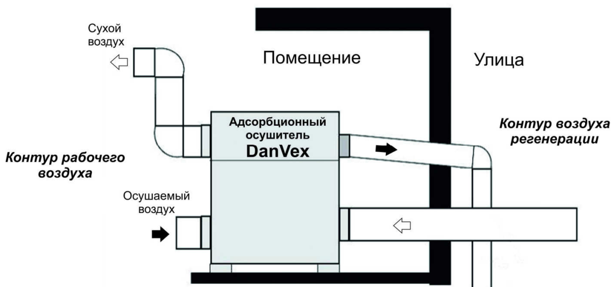
Основная схема установки адсорбционного осушителя DanVex
