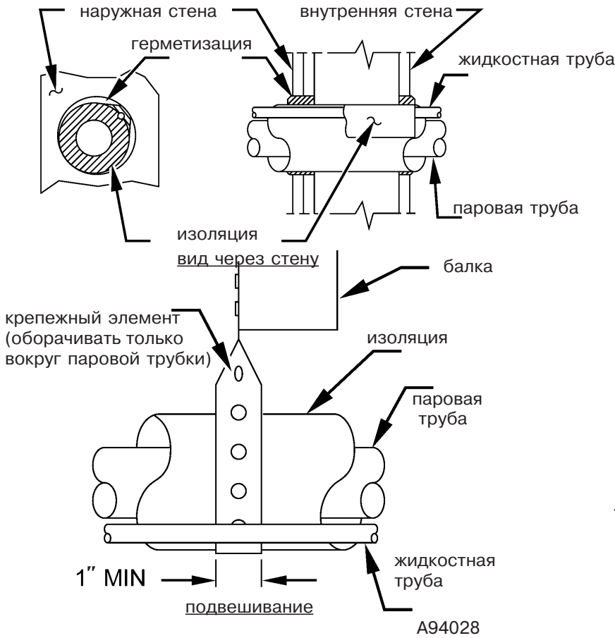
Рис. 3 - Подсоединение фреонпроводов
